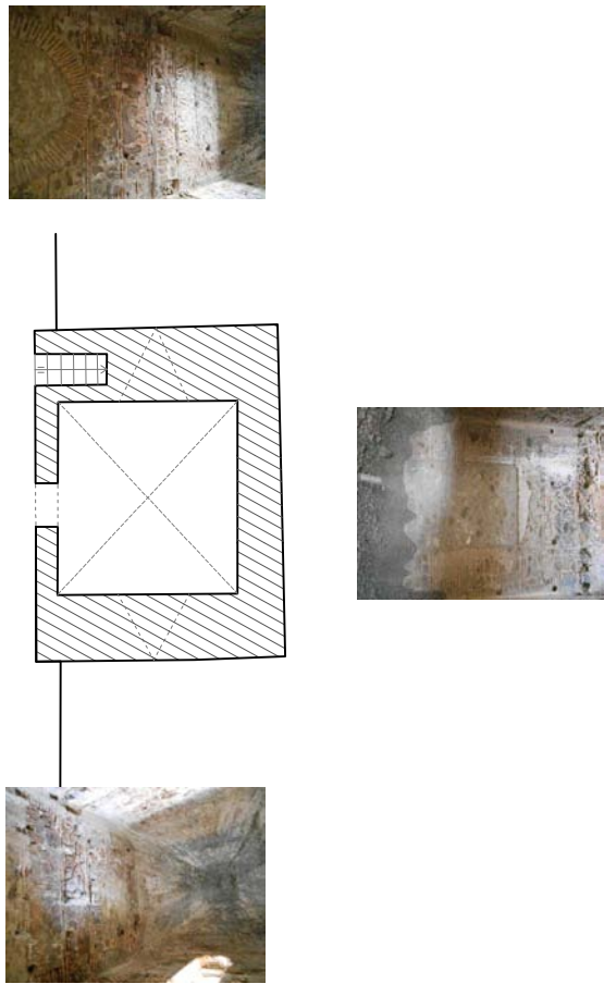
SECCIÓN DD'
