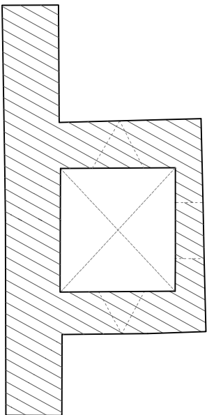
SECCIÓN CC'
