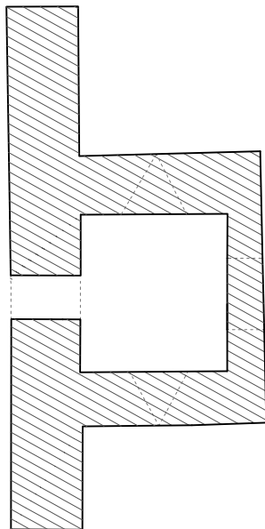
SECCIÓN BB'
